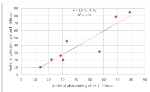
Figur 1. Sammenhæng mellem andel af afstrømning, der sker efter 1. februar og den tilhørende udvaskning
